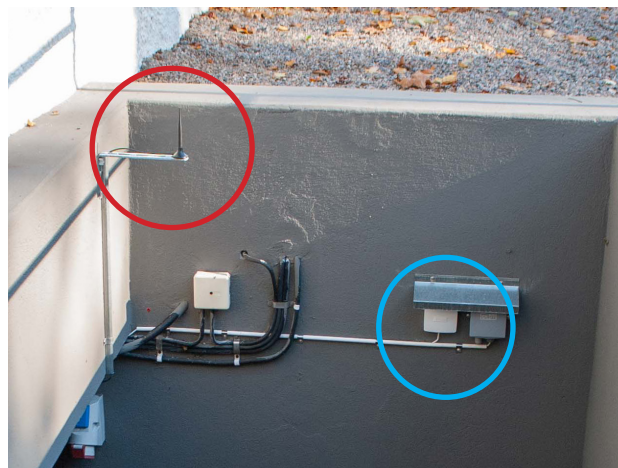
En sändare sitter ovanför dörren till pannrummet i källaren, röd ring. På väggen intill sitter också utomhusgivaren, blå ring.
